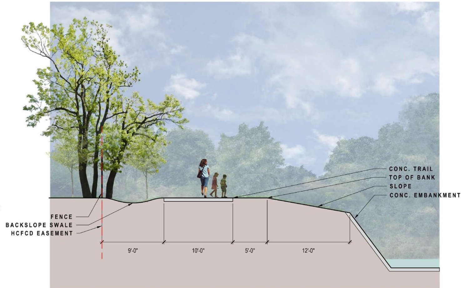
TRAIL AT BACKSLOPE SWALES SENDERO CON DRENAJE CENEGAL A UN COSTADO
